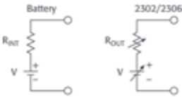
Упрощенная эквивалентная схема батареи и источника питания 2302/2306.
